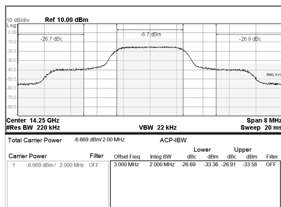
P_{OUT}=37\text{dBm} IDQ=2.45\text{A}
